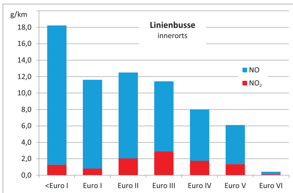
Abbildung 2: \text{NO}_x - und \text{NO}_2 -Emissionsfaktoren (innerorts) von Diesel-Linienbussen.
